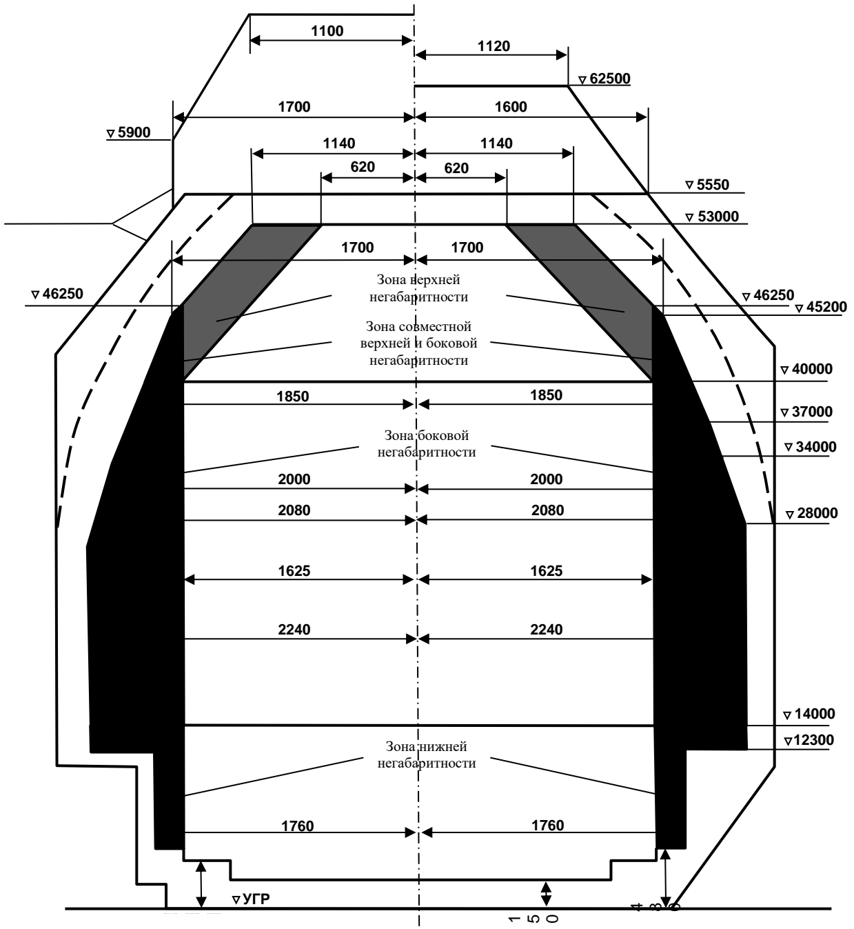
Рис.1. Зоны негабаритности груза
